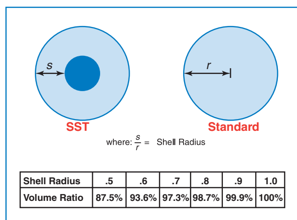
Fig. 2 Diffusion Path
