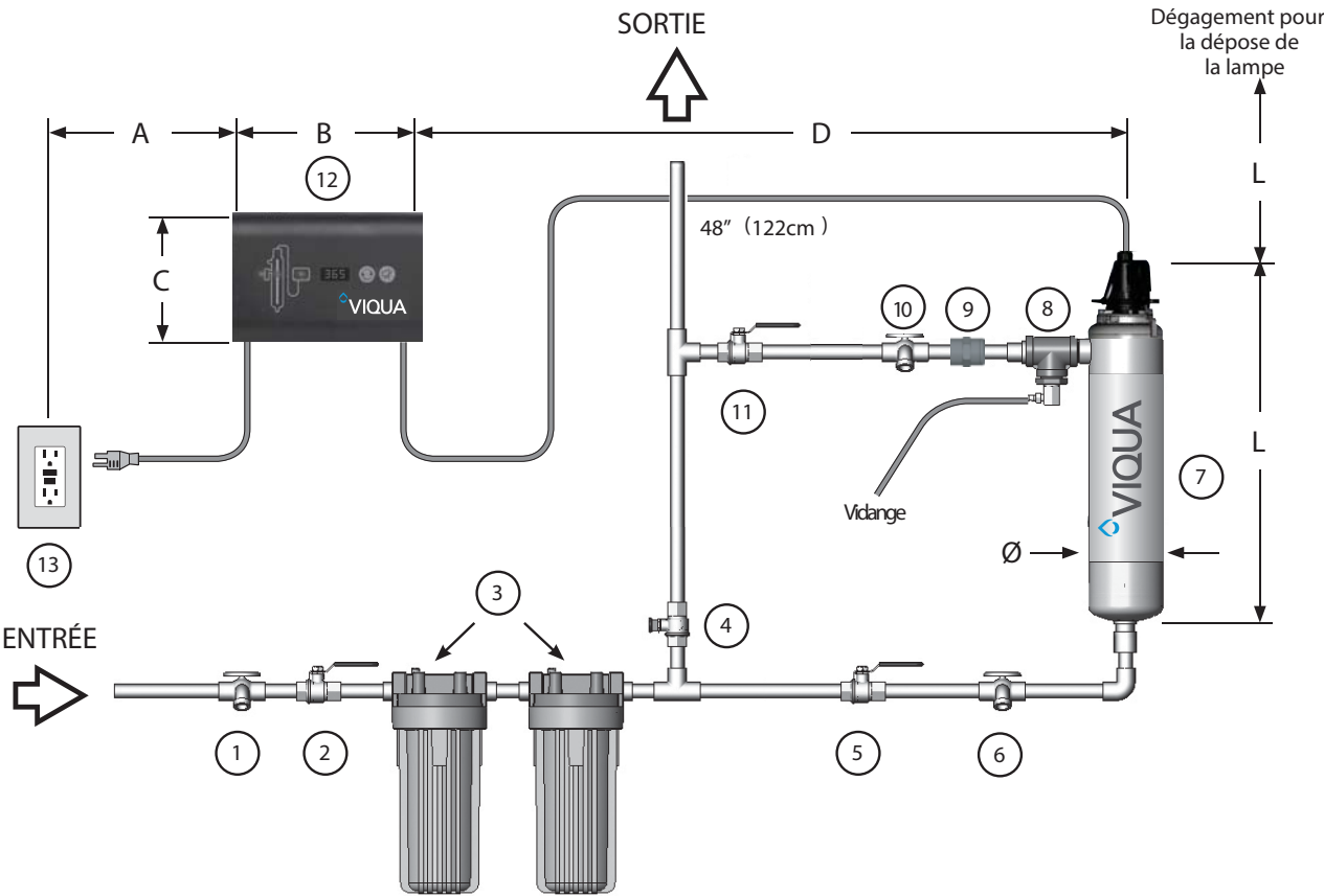
Figure 3 Système - Dimension et agencements
