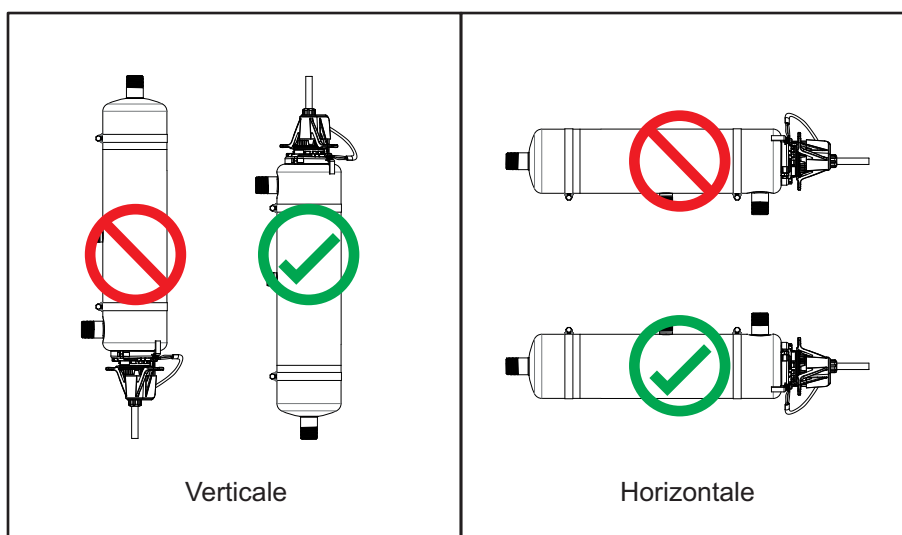
Figure 4 Installation du système de désinfection - Verticale et Horizontale
